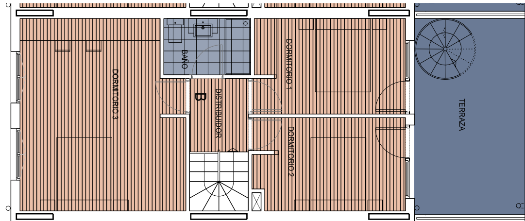
PLANTA PRIMERA
